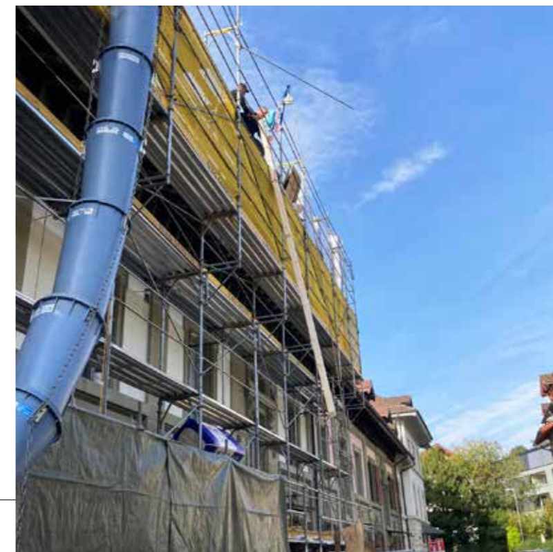
Dachsanierung am Pavillonweg in Bern.
